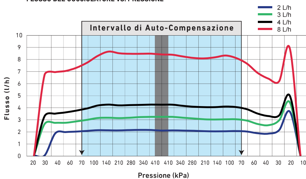
FLUSSO DEL GOCCIOLATORE VS. PRESSIONE
