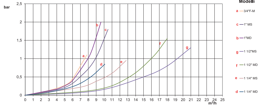
Grafico perdite di carico filtri M
